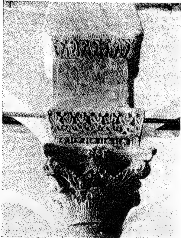
(شكل ١٥) قرم وطنوف حجرية في المجنبة التي تلى بيت الصلاة
